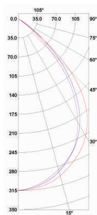
Zenith F1 2x36W
